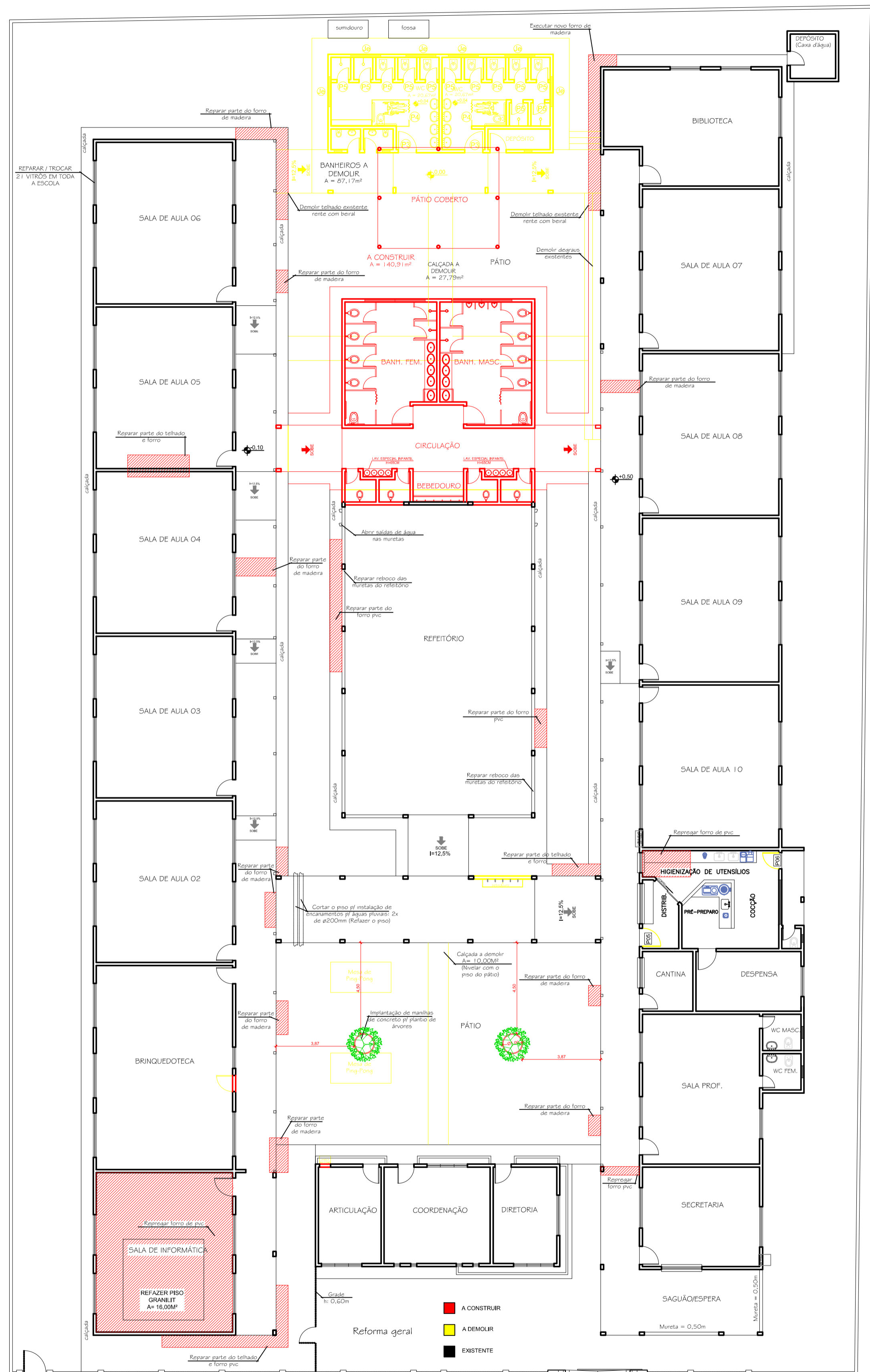
PLANTA CONSTRUÇÃO/DEMOLIÇÃO ESC. 1:150
