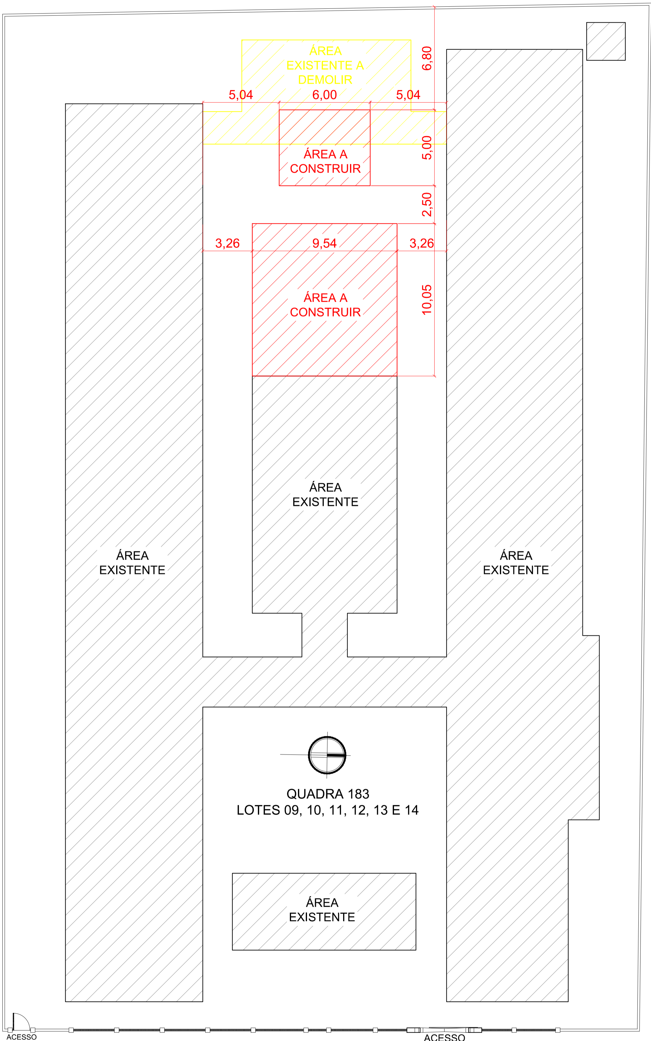
IMPLANTAÇÃO ESC. 1:150
